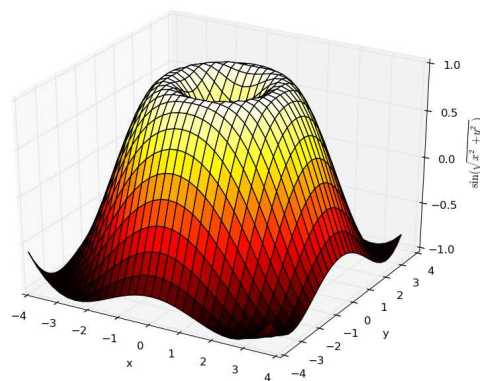
Figura 8: Gráfico 3D da superficie z = \sin \sqrt{x^2 + y^2} .
