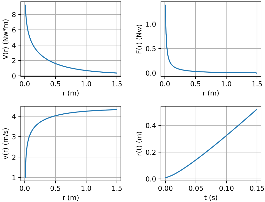
Figura 7: Potencial V(r) , forza F(r) , velocidade v(r) e radio r(t) no exercicio do potencial.
